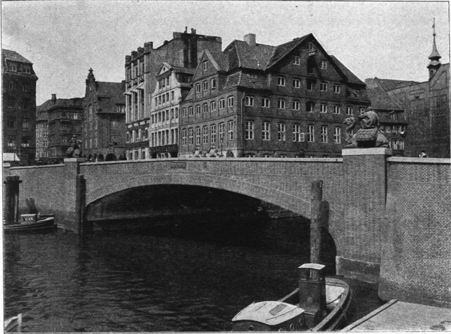
Abb. 283. Schaartorbrücke, Ansicht.
