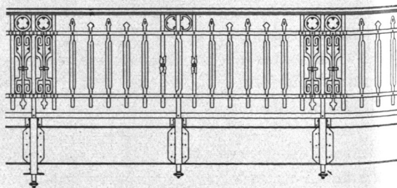
Abb. 280. Wandrahmsbrücke, Einzelheiten des Geländers.
