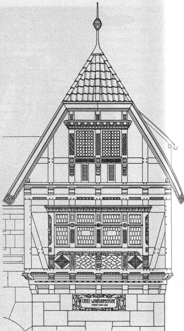
Abb. 278. Wandrahmsbrücke, Einzelheiten des Giebels am Meßberg.
