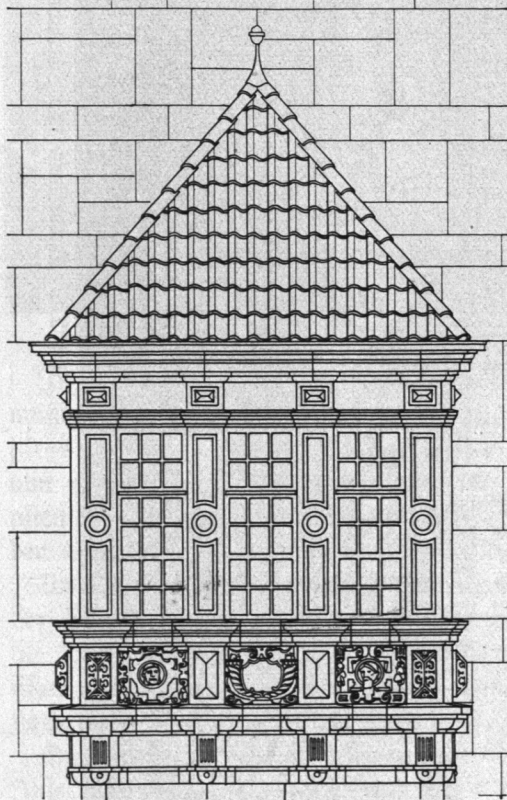
Abb. 279. Wandrahmsbrücke, steinerner Erker am Meßberg.
