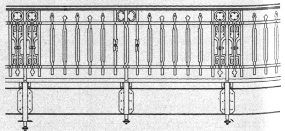
Abb. 280. Wandrahmsbrücke, Einzelheiten des Geländers.
