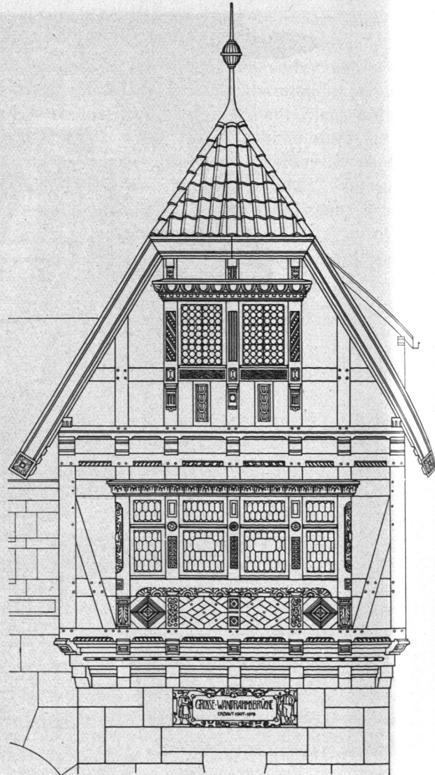
Abb. 278. Wandrahmsbrücke, Einzelheiten des Giebels am Meßberg.
