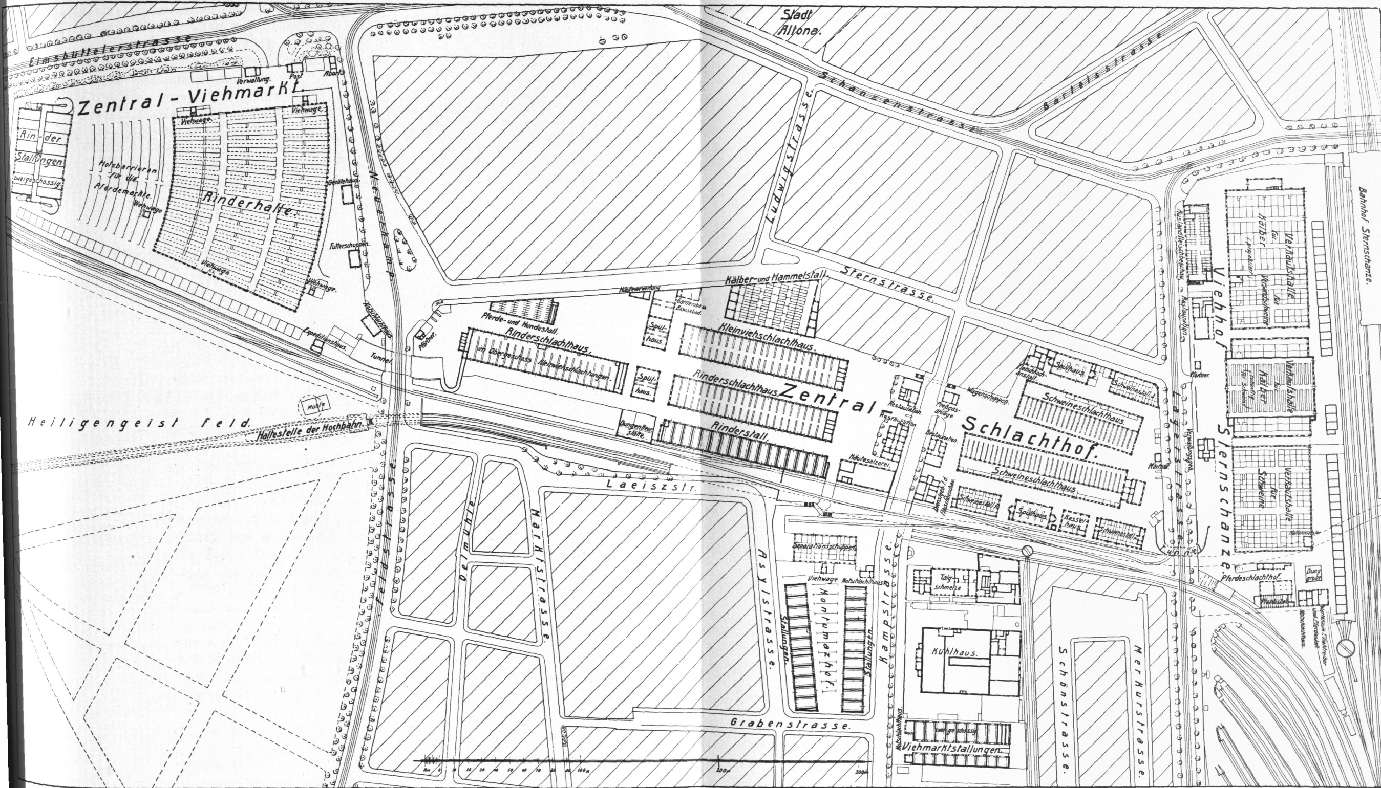
Lageplan des Zentral-Viehmarktes und Schlachthofes.
