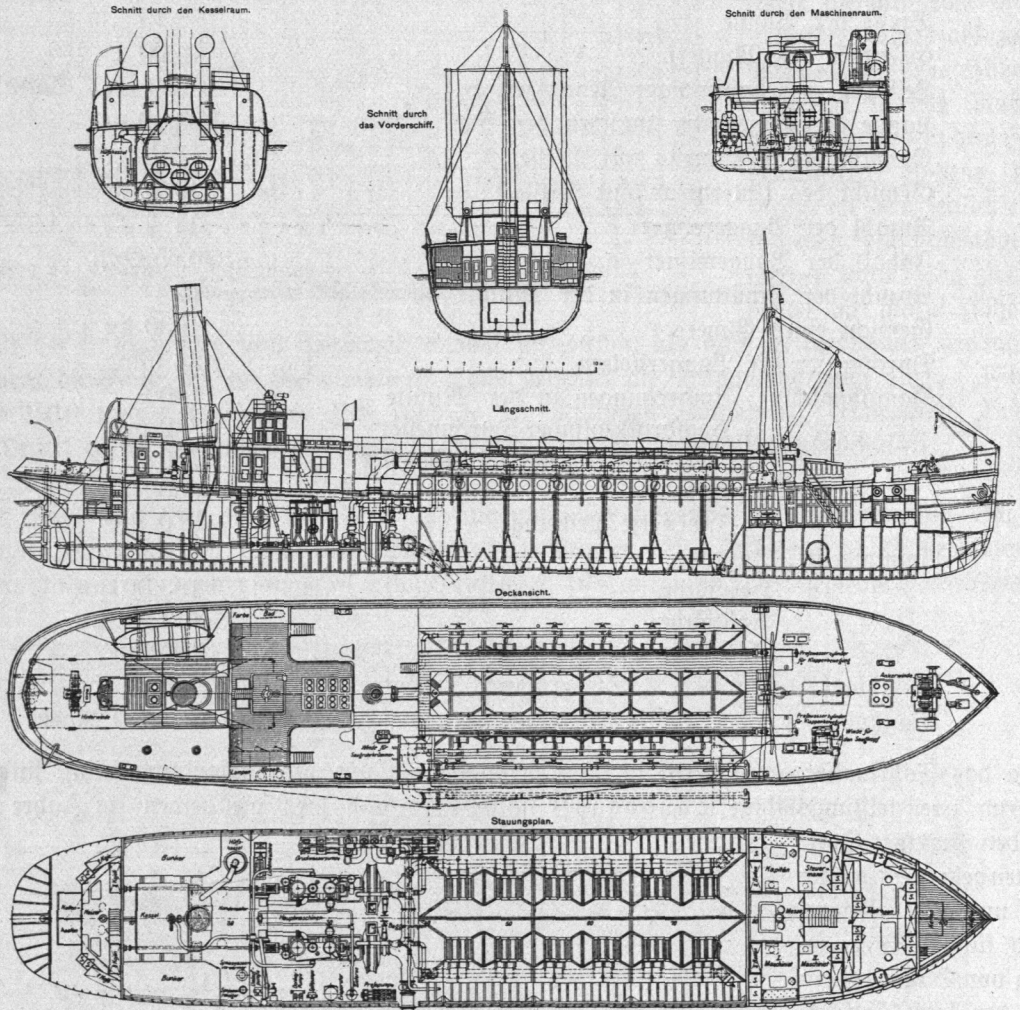
Abb. 26 bis 31. Bauart des Saugbaggers XV.
