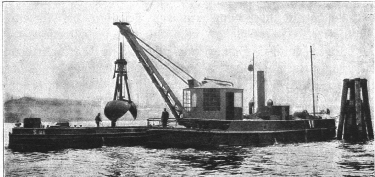
Abb. 33. Greifbagger VI.
