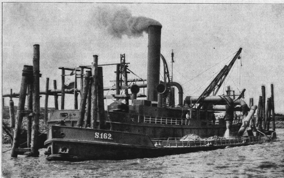
Abb. 38. Schutensauger IV.
