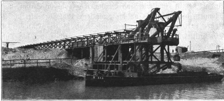
Abb. 22. Hängebahn.
