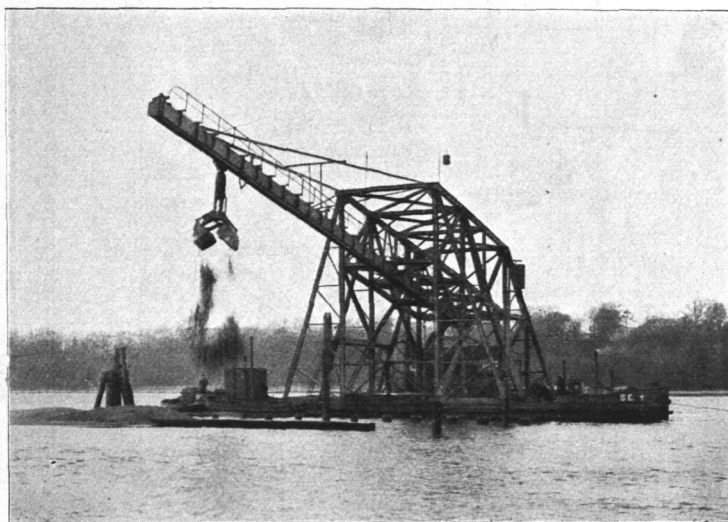
Abb. 42. Schutenentleerer II.
