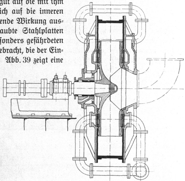
Abb. 39. Baggerpumpe.
