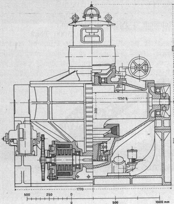
Abb. 44. Schiffskreisfel, Peildampfer „Schaarhorn“.
