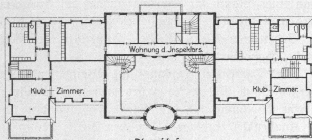
Obergeschoß.
