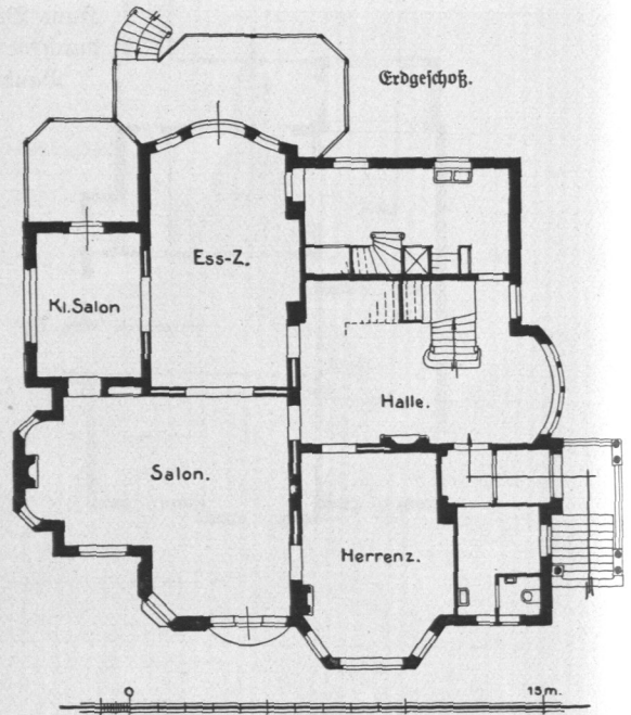
Abb. 1008 und 1009. Haus C. von Boje, Maria-Louisen-Strasse 39, erbaut 1900 durch die Architekten B. D. A. Lundt & Kallmorgen. Baukosten 110 000 Mark.
