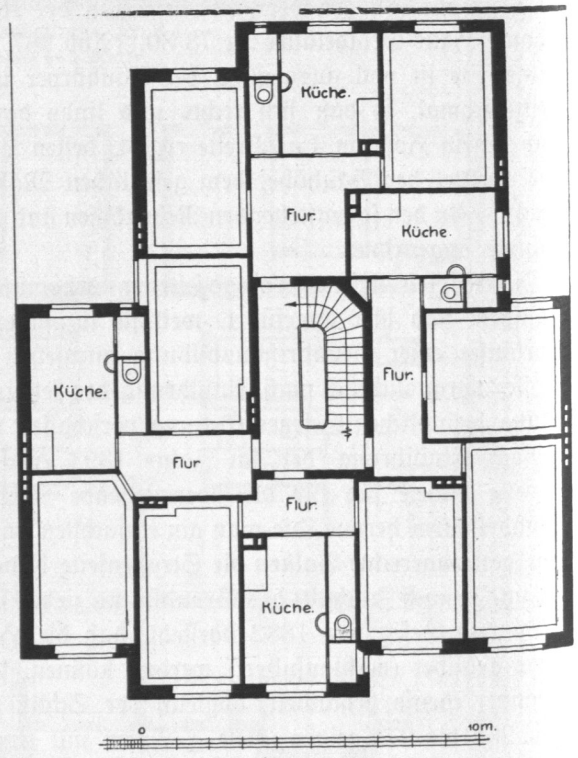
Abb. 971. Haus Dulsberg Nr. 2, Obergeschoß.
