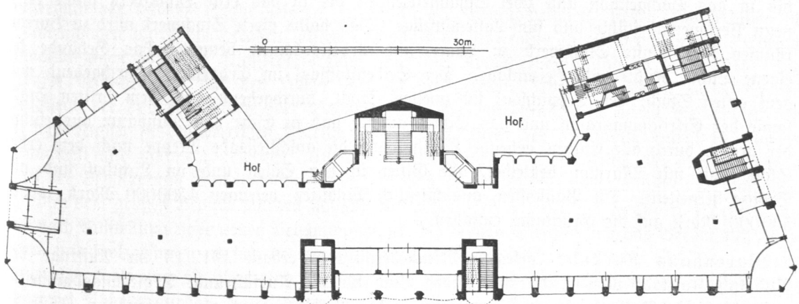
Abb. 940. Warenhaus Karstadt, Erdgeschoß.
