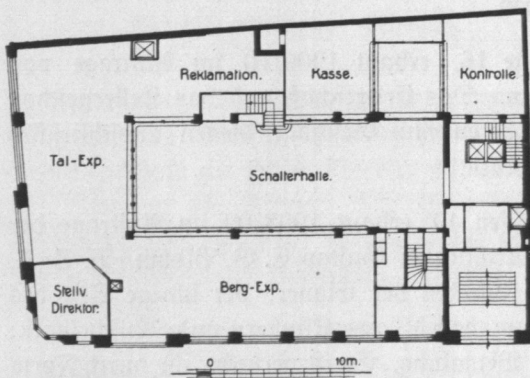
Abb. 880. Haus Elbeschiffahrt, Erdgeschöß.
