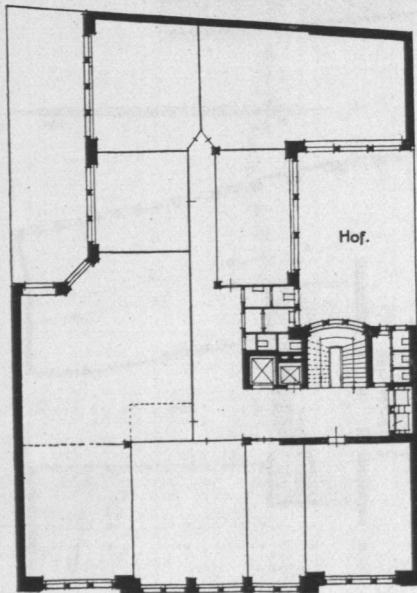
Abb. 867. Caledoniahaus, Grundriß.
