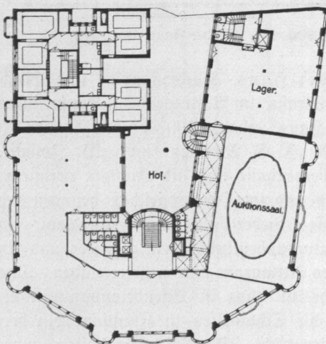
Abb. 848. Fruchthof, Grundriß.
