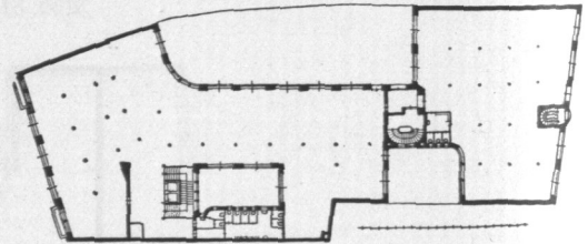
Abb. 820. Elbhof, Grundriß.
