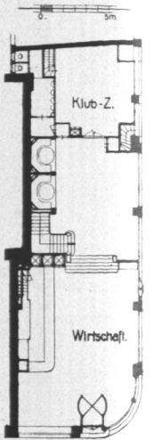
Abb. 765. Restaurant Bagener, Erdgeschöß.
