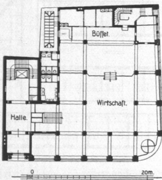
Abb. 743. Rathaus-Hotel, Erdgeschoss, Grundriß.
