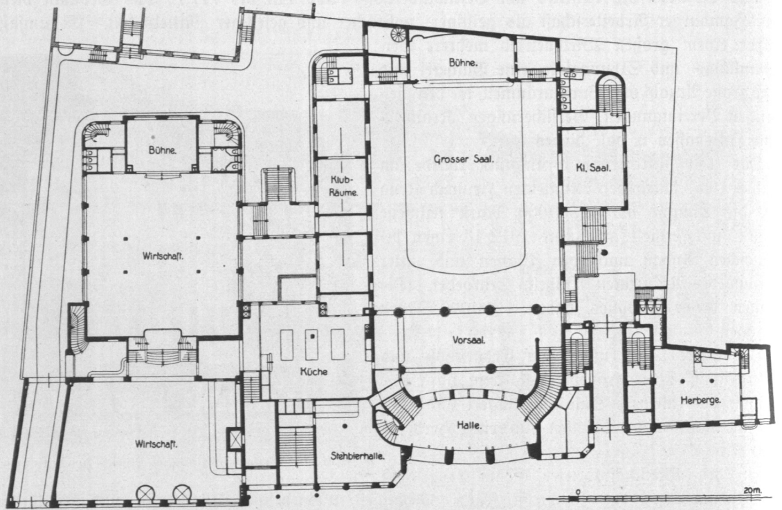
Abb. 716. Gewerkſchaftshaus, Erdgeſchoß, Grundriß.
