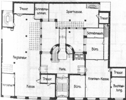
Abb. 710. Geschäftshaus des Vereins für Handlungs-Commis von 1858, Erdgeschoss, Grundriß.
