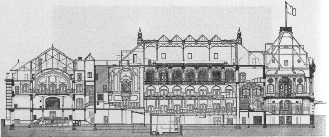
Abb. 673. Musikhalle, Längenschnitt.
