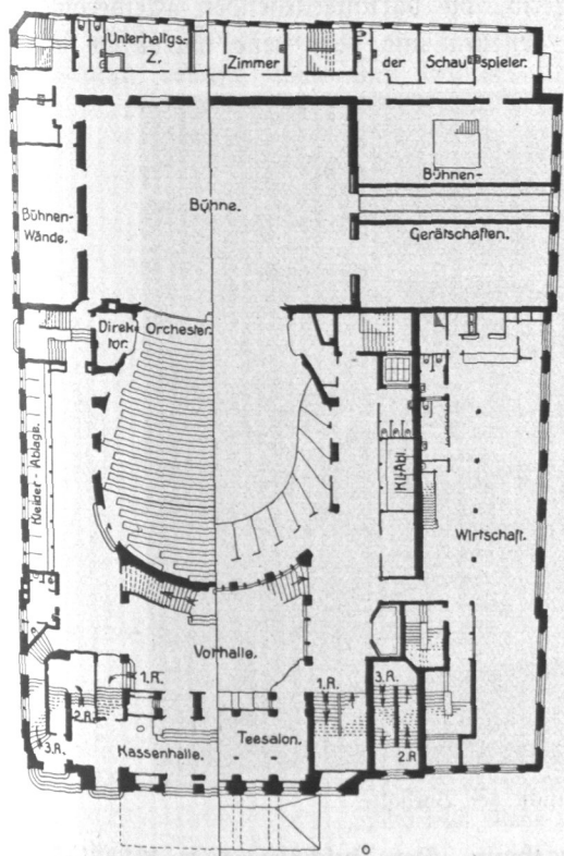
Abb. 644. Thaliatheater, Parkett- und Logenrang, Grundriß.
