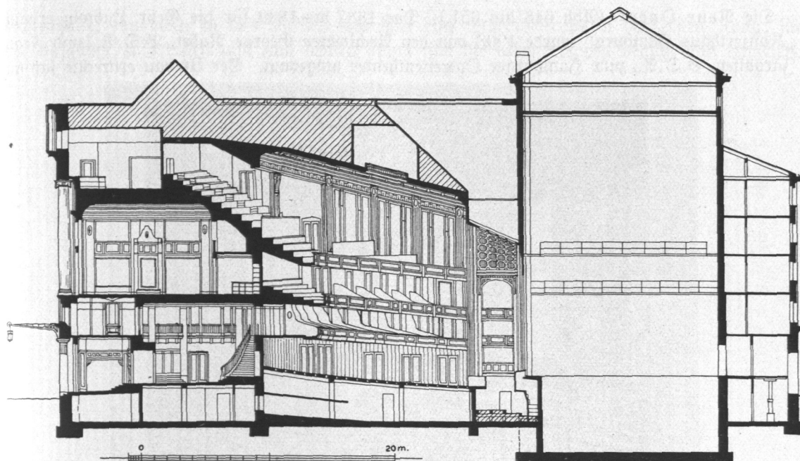
Abb. 643. Thaliatheater, Längenschnitt.
