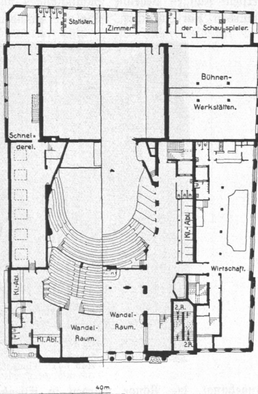
Abb. 645. Thaliatheater, 3. Rang und 1. Rang, Grundriß.
