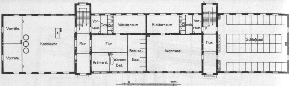
Abb. 628. Werk- und Armenhaus in Farmsen, großes Frauenhaus, Erdgeschoß, Grundriß.
