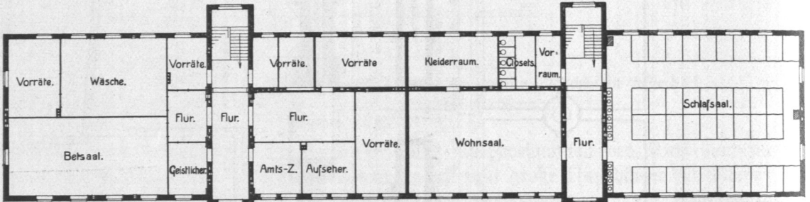
Abb. 629. Werk- und Armenhaus in Farmsen, großes Frauenhaus, Obergeschoß, Grundriß.
