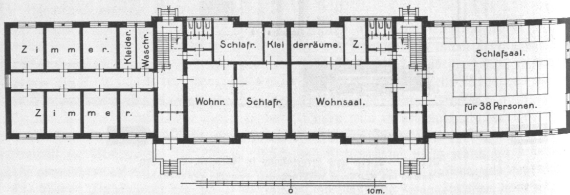
Abb. 631. Werk- und Armenhaus in Farmsen, großes Einzelhaus, Grundriß.
