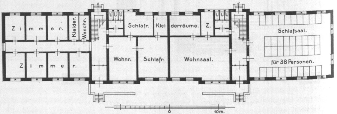
Abb. 631. Werk- und Armenhaus in Farmsen, großes Einzelhaus, Grundriß.
