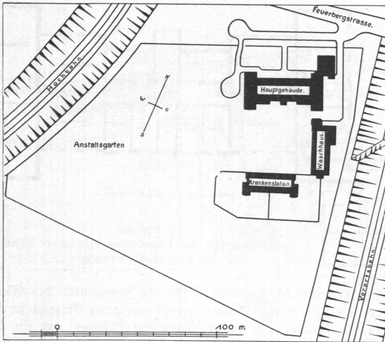
Abb. 624. Erziehungsanstalt für schulentlassene Mädchen in Alsterdorf, Lageplan.
