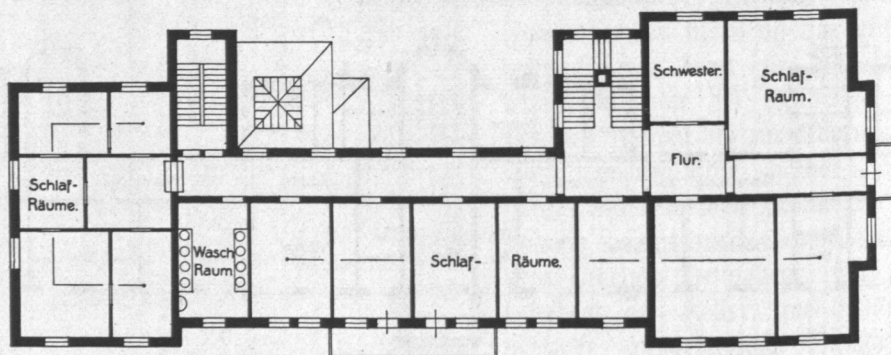
Abb. 619. Genesungs- und Erholungsheim Groß-Hansdorf, Gebäude für Frauen, Obergeschoß, Grundriß.
