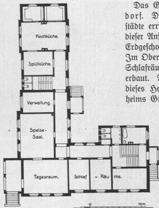
Abb. 617. Genesungs- und Erholungsheim Groß-Hansdorf, Gebäude für Kinder, Erdgeschoss, Grundriß.
