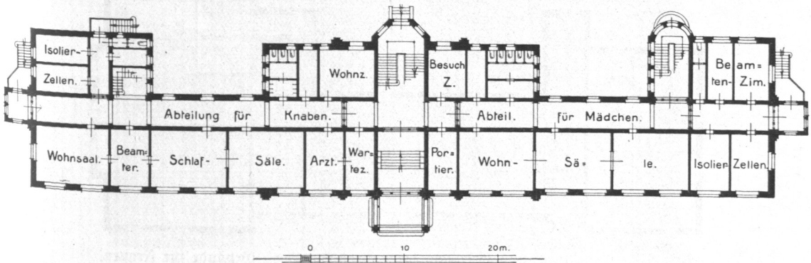
Abb. 616. Verwaltungsgebäude des Waisenhauses, Grundriß.
