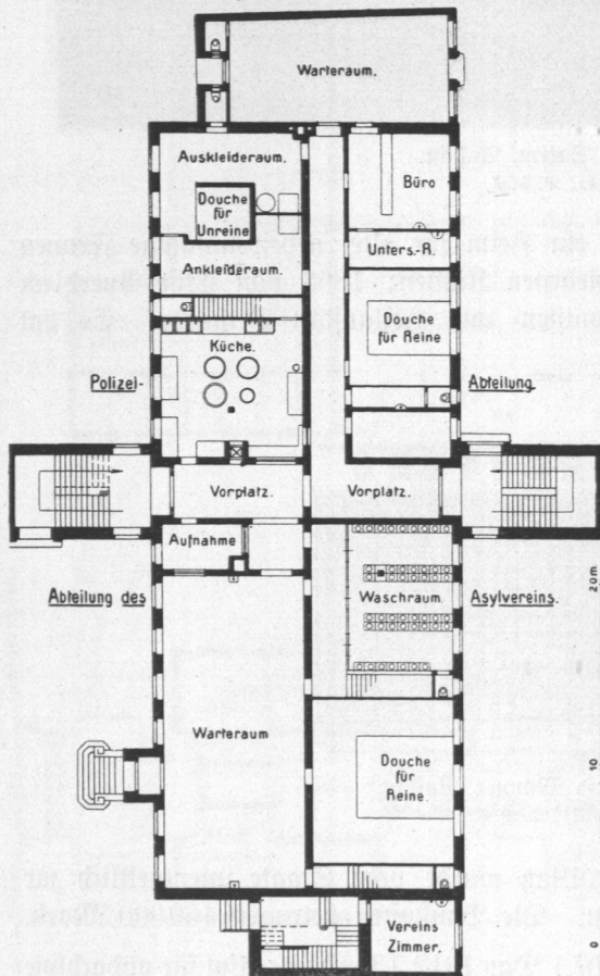
Abb. 606. Asyl für obdachlose Männer, Erdgeschoß, Grundriß.
