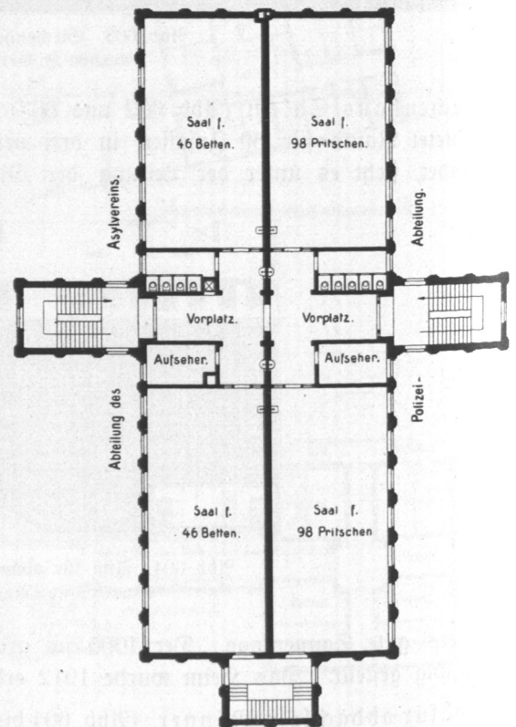
Abb. 607. Asyl für obdachlose Männer, Obergeschoß, Grundriß.
