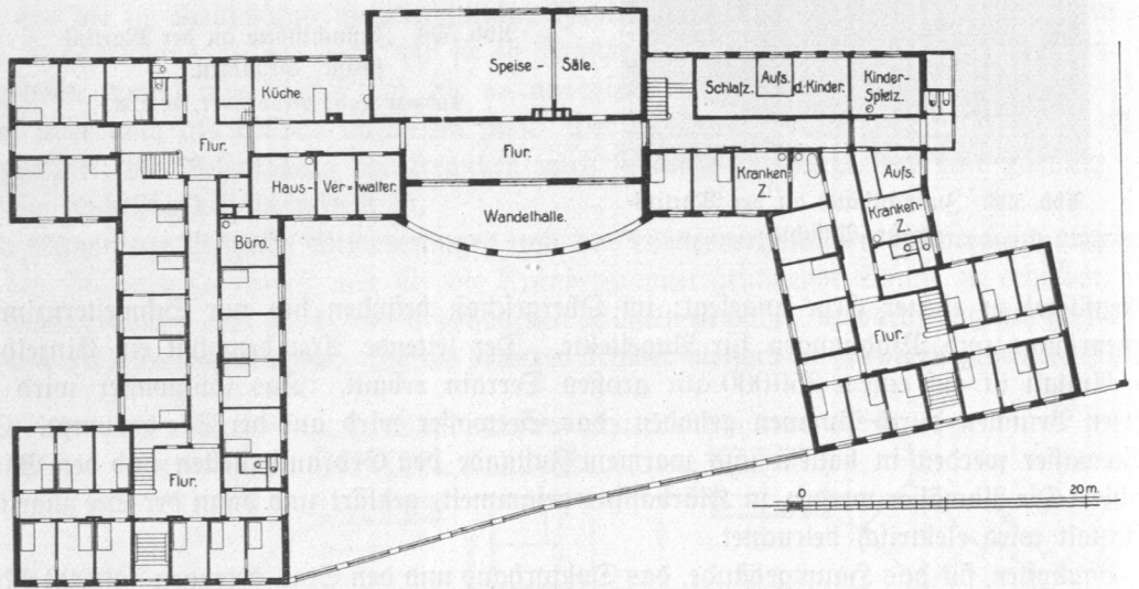
Abb. 601. Blinden-Asyl, Grundriß.
