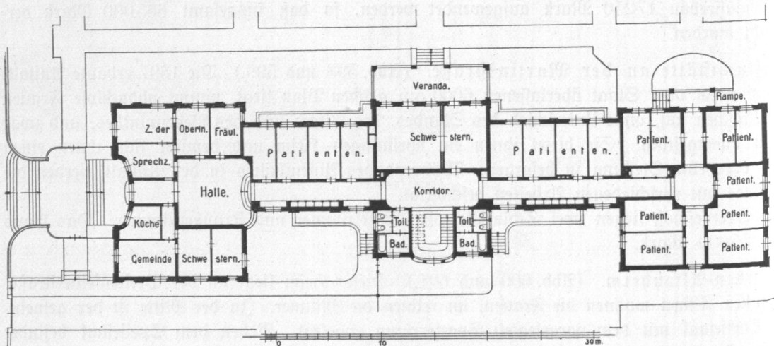
Abb. 602. Sieschenhaus Salem, Grundriß.
