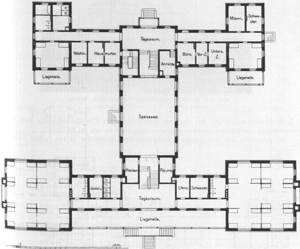
Abb. 588. Heilstätte Edmundsthal, Thekla-Haus, Grundriß.
