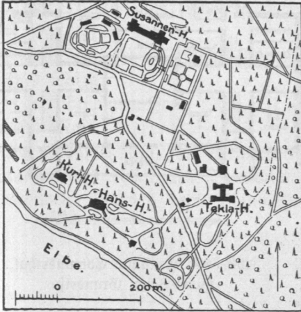
Abb. 586. Heilstätte Edmundsthal, Lageplan.
