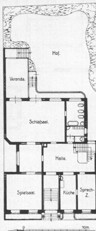
Abb. 544. Kinderbewahranstalt von 1852, Erdgeschoß, Grundriß.
