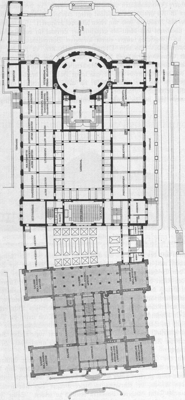
Abb. 508. Kunstihalle, Erdgeschoss, Grundriß.
