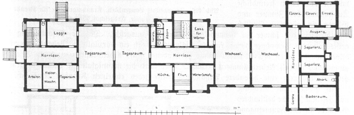
Abb. 494. Irrenanstalt Langenhorn, Überwachungshaus für 50 Männer und 8 Wärter, Erdgeschöß, Grundriß.
