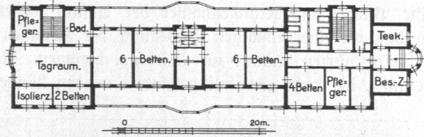
Abb. 482. Irrenanstalt Friedrichsberg, Haus für unruhige Männer IV. Klasse, Erdgeschoß, Grundriß.
