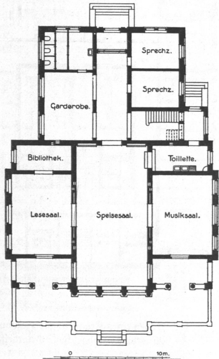
Abb. 445. Allgemeines Krankenhaus Hamburg-Barmbeck, Schwesternhaus, Erdgeschoß, Grundriß.
