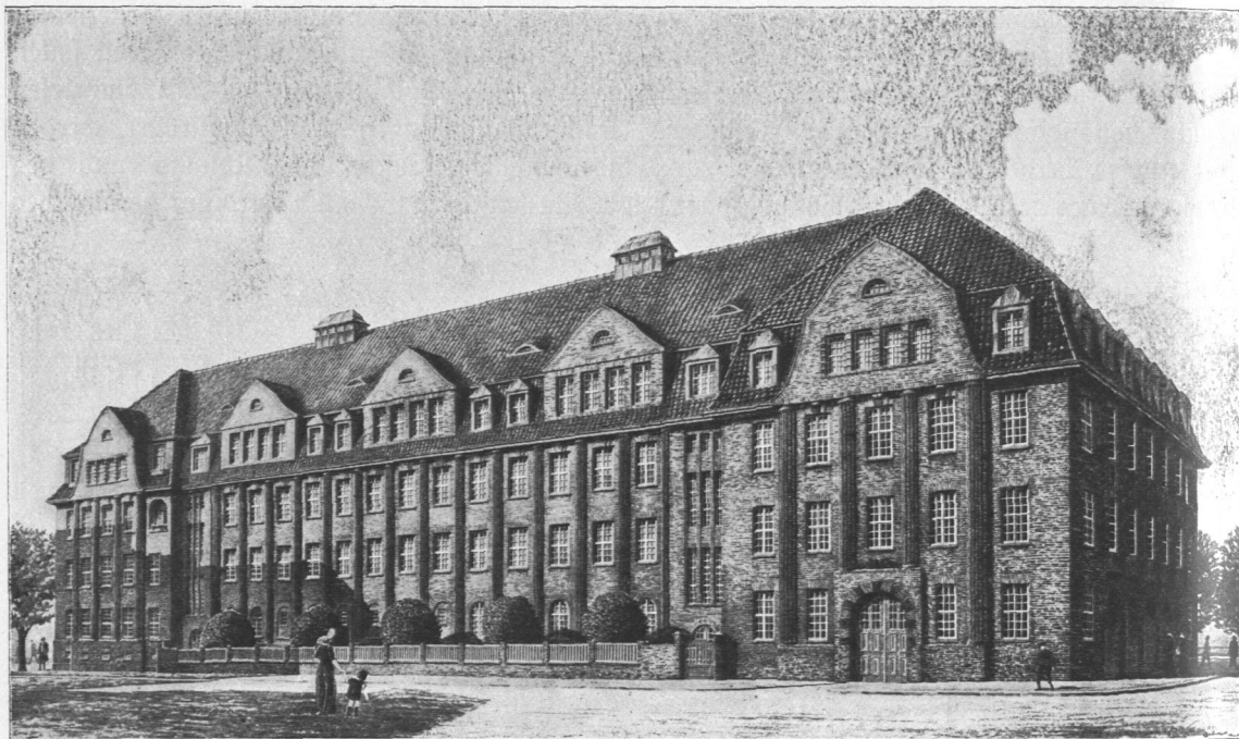
Abb. 396. Hauptfeuerwache am Berliner Tor, Ansicht. Entwurf: Baudirektor Professor Schumacher.
