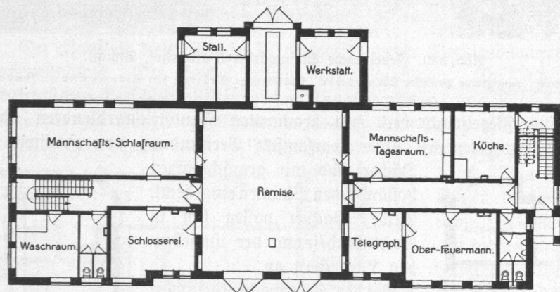
Abb. 393. Feuerwache Ecke Alsterkrugchauffee-Maienweg, Erdgeschoss.
