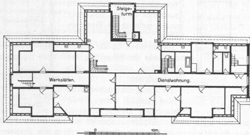
Abb. 394. Feuerwache Ecke Alsterkrugchauffee-Maienweg, Obergeschoss.
