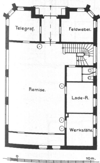
Abb. 390. Feuerwache Steinwärder-Waltershof, Erdgeschoss.
