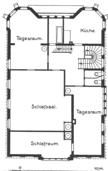
Abb. 391. Feuerwache Steinwärder-Waltershof, Obergeschoss.
