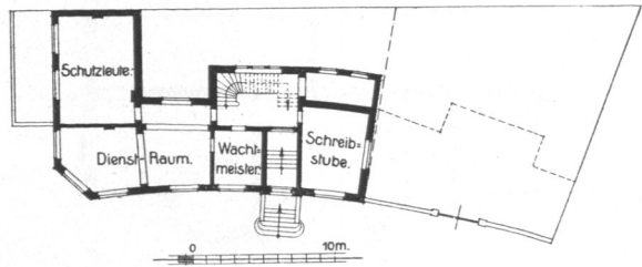
Abb. 352. Polizeiwache Hammerdeich, Erdgeschoß, Grundriß.
