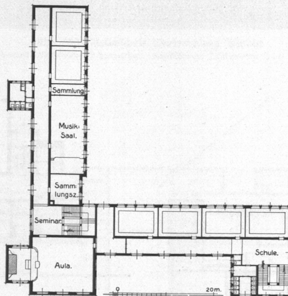
Abb. 239. Lehrerinnenseminar an der Hohen Weide, Obergeschoß.
