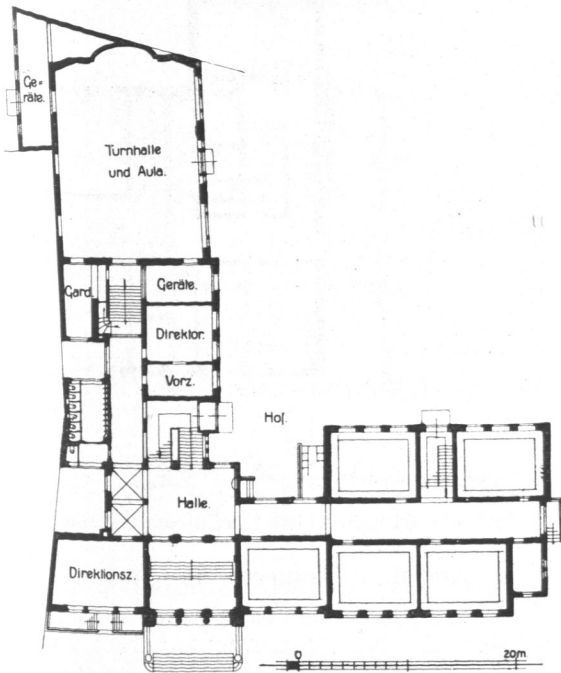
Abb. 296. Talmud-Tora-Schule, Grundriß, Erdgeschoß.
