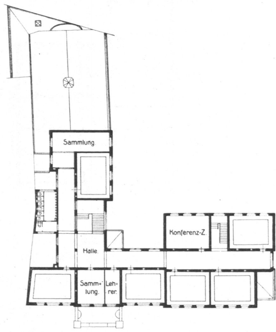
Abb. 297. Talmud-Tora-Schule, Grundriß, Obergeschoss.
