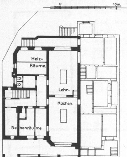
Abb. 293. Haushaltungsschule Wallstraße, Kellergrundriß.
