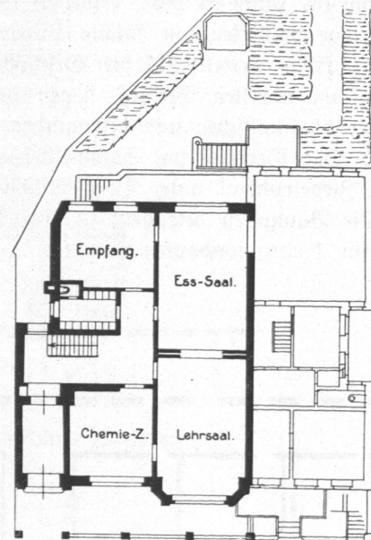
Abb. 294. Haushaltungsschule Wallstraße, Erdgeschoss.
