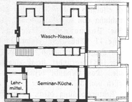
Abb. 292. Haushaltungsschule Wallstraße, Dachgeschoss.
