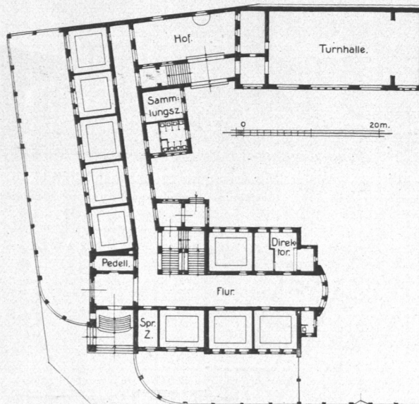
Abb. 287. Höhere Mädchenschule Hansastraße, Erdgeschoss.
