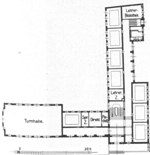
Abb. 278. Realschule Bogenstraße, Erdgeschoss.
