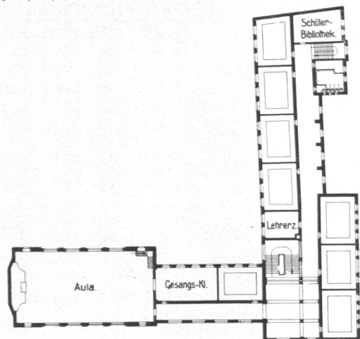
Abb. 279. Realschule Bogenstraße, Obergeschoss.
