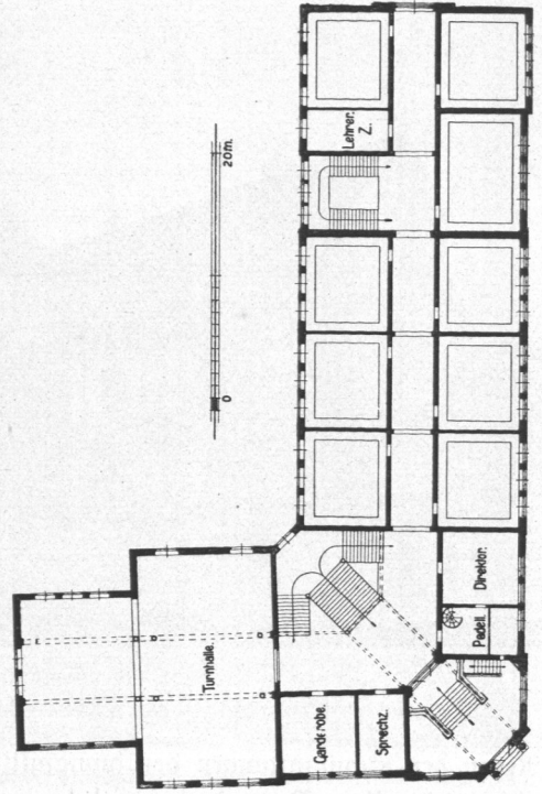
Abb. 272. Oberrealschule Iwerhoffstraße, Erdgeschoss.
