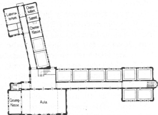
Abb. 264. Realgymnasium Kaiser-Friedrich-Upper, Obergeschoss.
