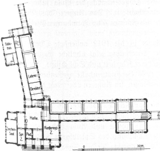
Abb. 263. Realgymnasium Kaiser-Friedrich-Upper, Erdgeschoss.
