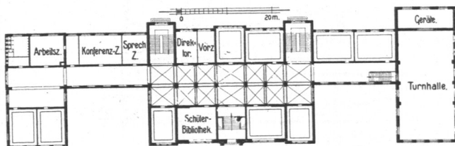
Abb. 258. Realgymnasium Armgartstraße, Erdgeschoß. Entwurf: Baudirektor Zimmermann.
