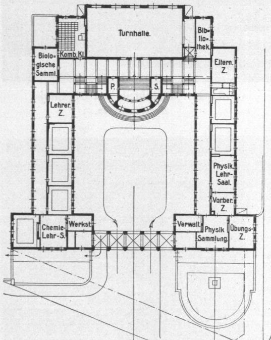
Abb. 255. Gelehrten Schule des Johanneums, Erdgeschoß.
