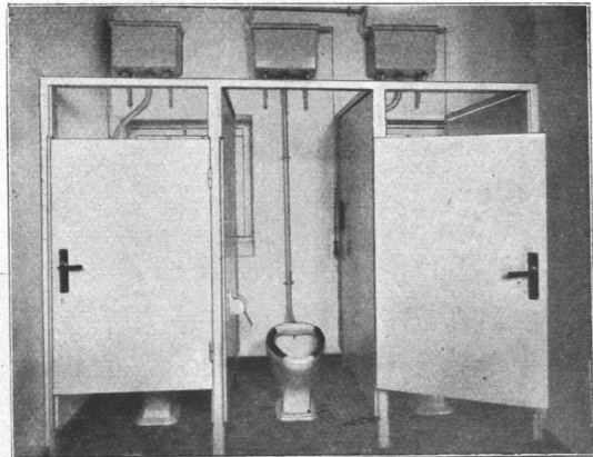
Abb. 241. Volksschule Forsmannstraße, Abortanlage.
