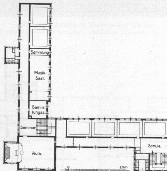
Abb. 239. Lehrerinnenseminar an der Hohen Weide, Obergeschoß.
