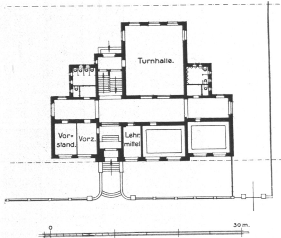
Abb. 237. Hilfsschule in der Finkenau, Erdgeschoß. Entwurf: Bauinspektor Dr. Ing. Erbe. Ausführung: Baurat Bauer.
