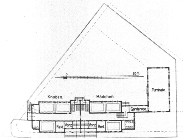
Abb. 236. Volksschule Tieloh, Erdgeschoß.
